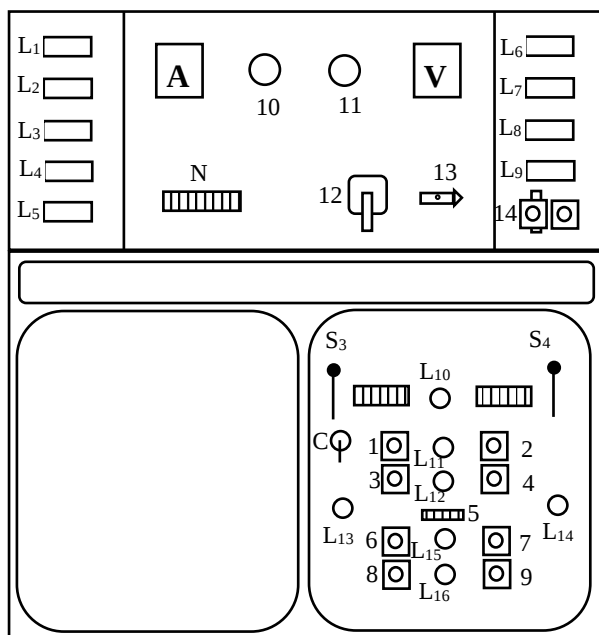
Fig. 10 – Pupitrul de comandă al instalației 250 kV, 50 Hz
